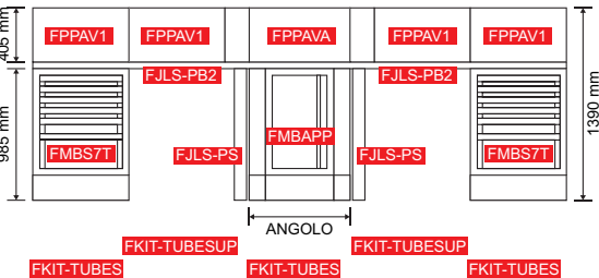
Schema di montaggio
