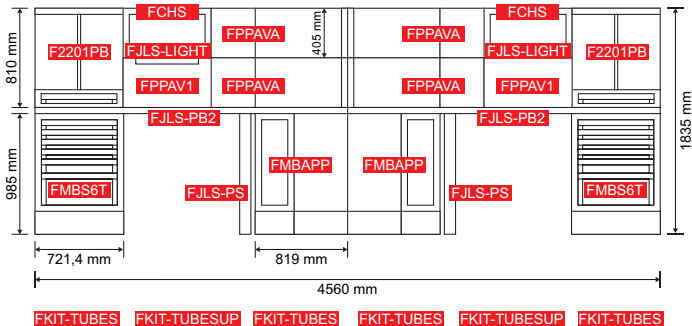
Schema di montaggio
